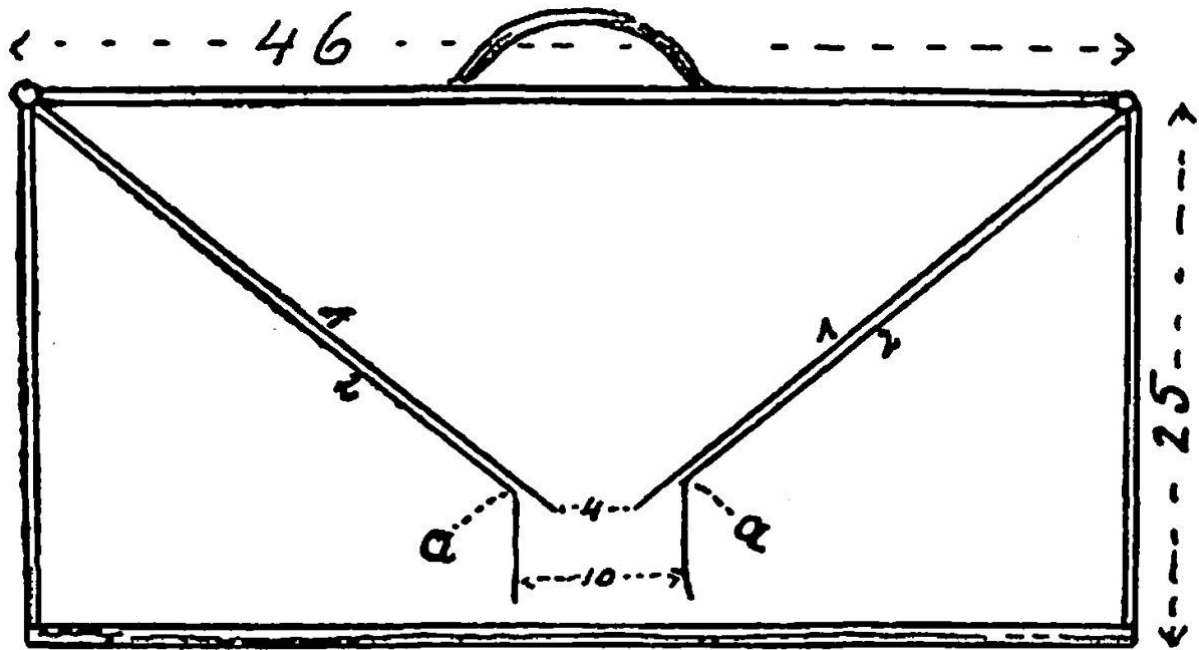
Verébfogóvarsa keresztmetszete.
